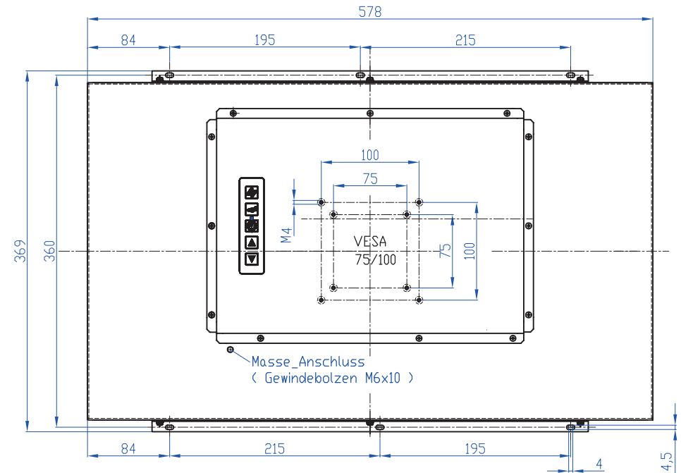
RÜCKANSICHT
