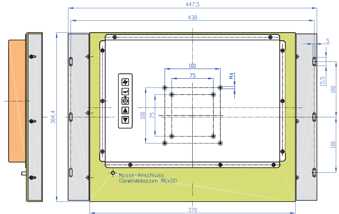
RÜCKANSICHT
